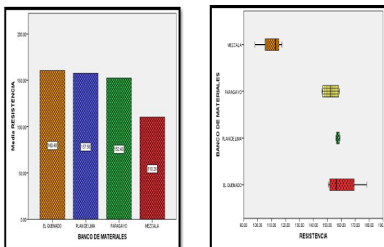
Figura 1 Comparación de la media de resistencia por banco
